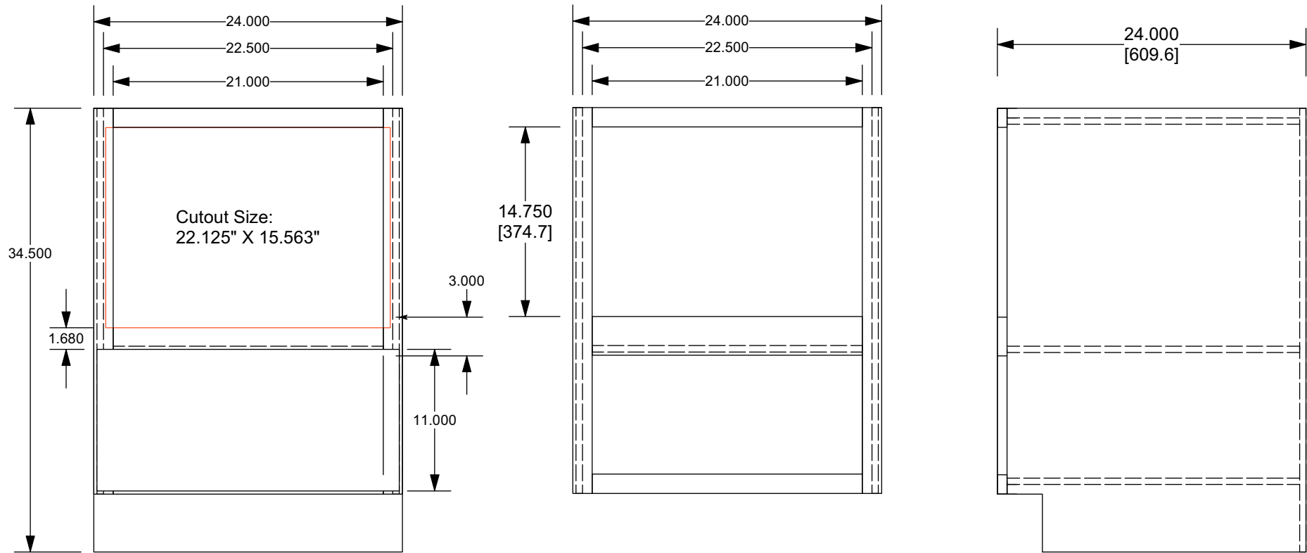
Elevation
